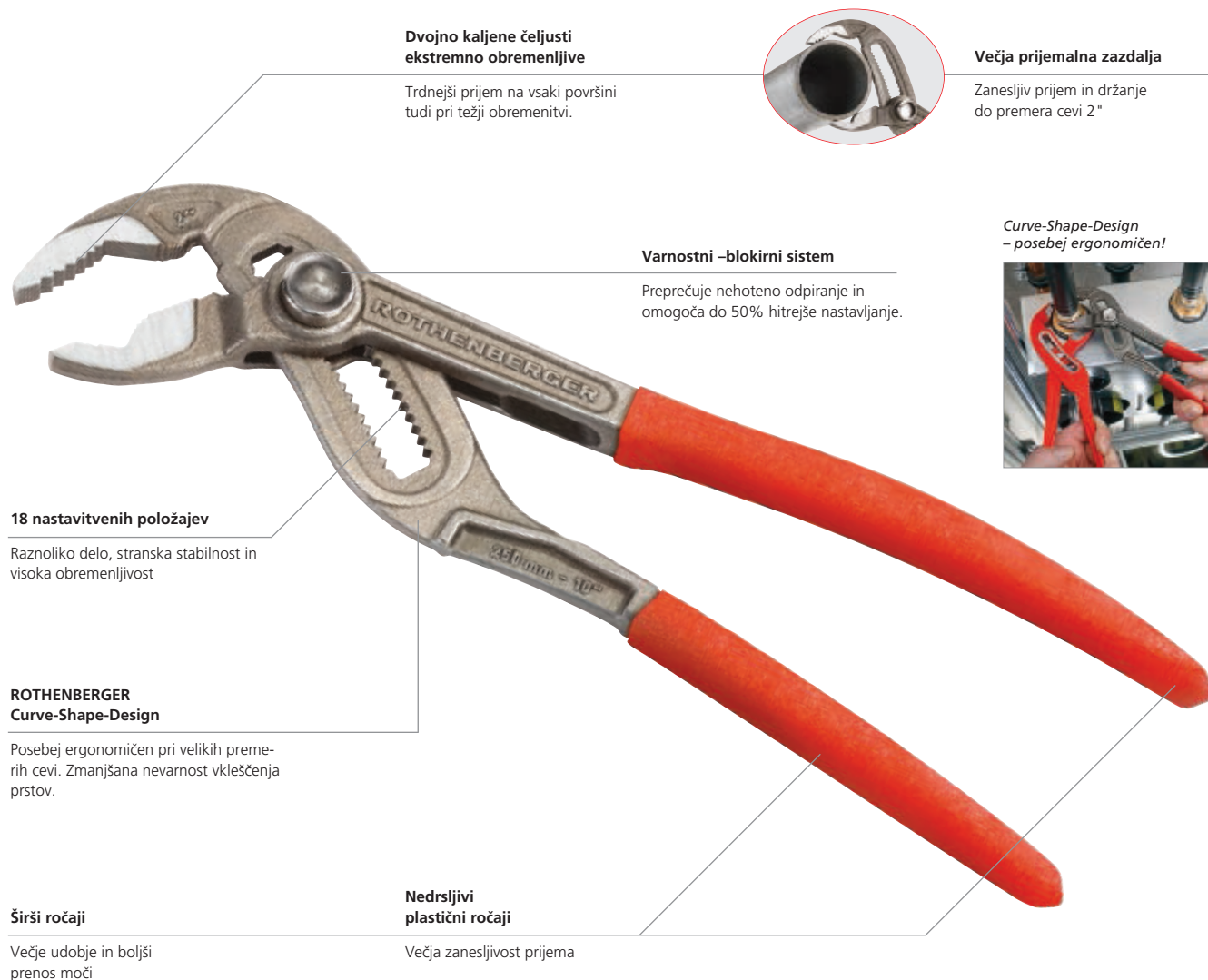
3-Točkovni prijem čez sredino za zanesljiv oprijem. Odličen prijem pri ceveh do Ø 2"
