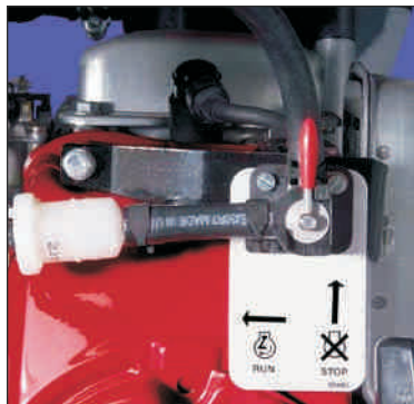
Kombinirano stikalo za zaprtje dovoda goriva in prekinitev tokokroga.
